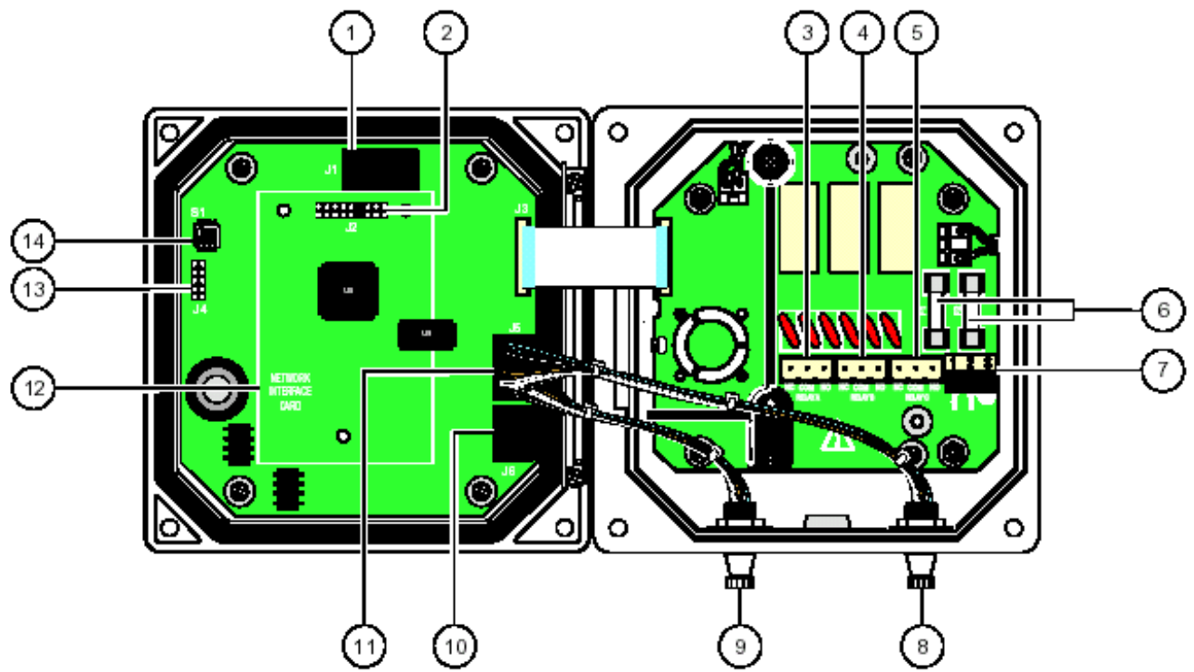
图 15 布线连接
